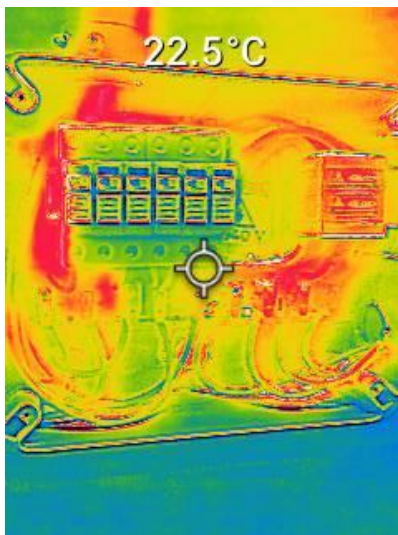
Figura 33 – Imagem com a câmera térmica da stringbox do inversor 1.
