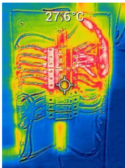
Figura 35 – Imagem com a câmera térmica do quadro principal da conexão CA.
